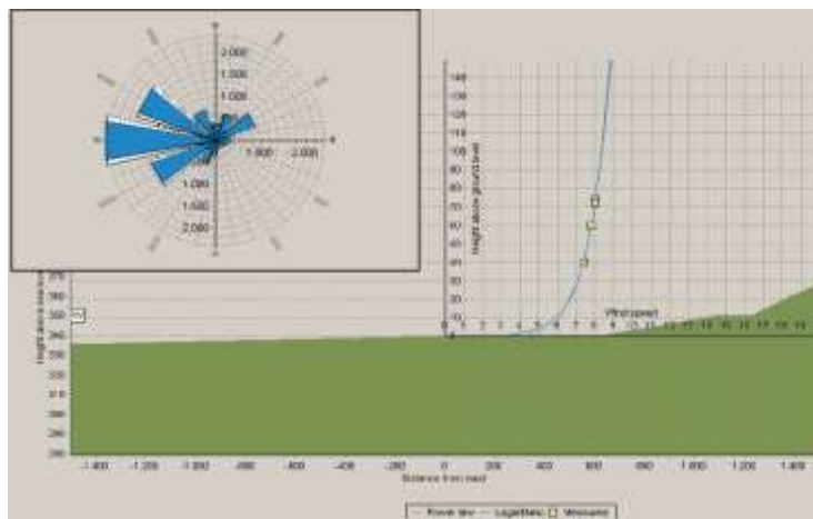
Figura 18. Distribución de las velocidades medias de viento y de dirección medidas a 72 metros. Fuente. ENAT SA
