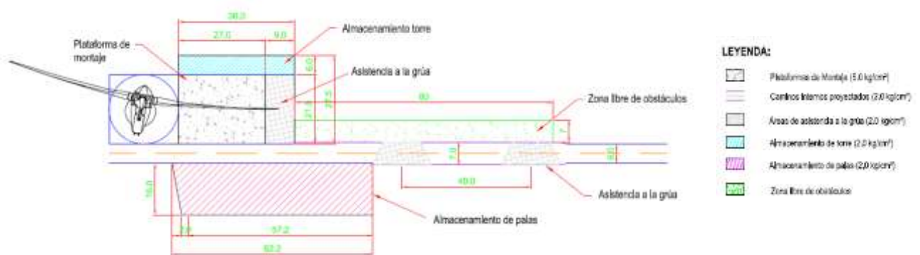
Figura 4. Configuración básica de áreas de maniobra
