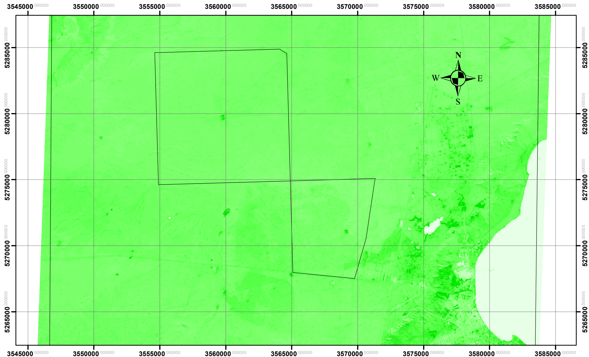
Figura 2 : Vegetación del área según índice verde (NDVI)
