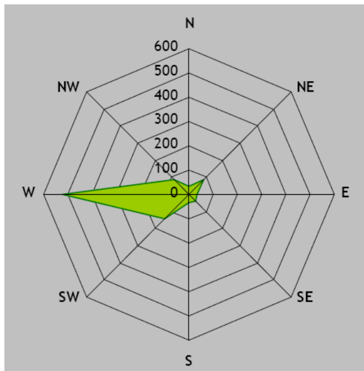
Figura 02. Rosa de los vientos Fuente. Scudelati & Asociados SA
