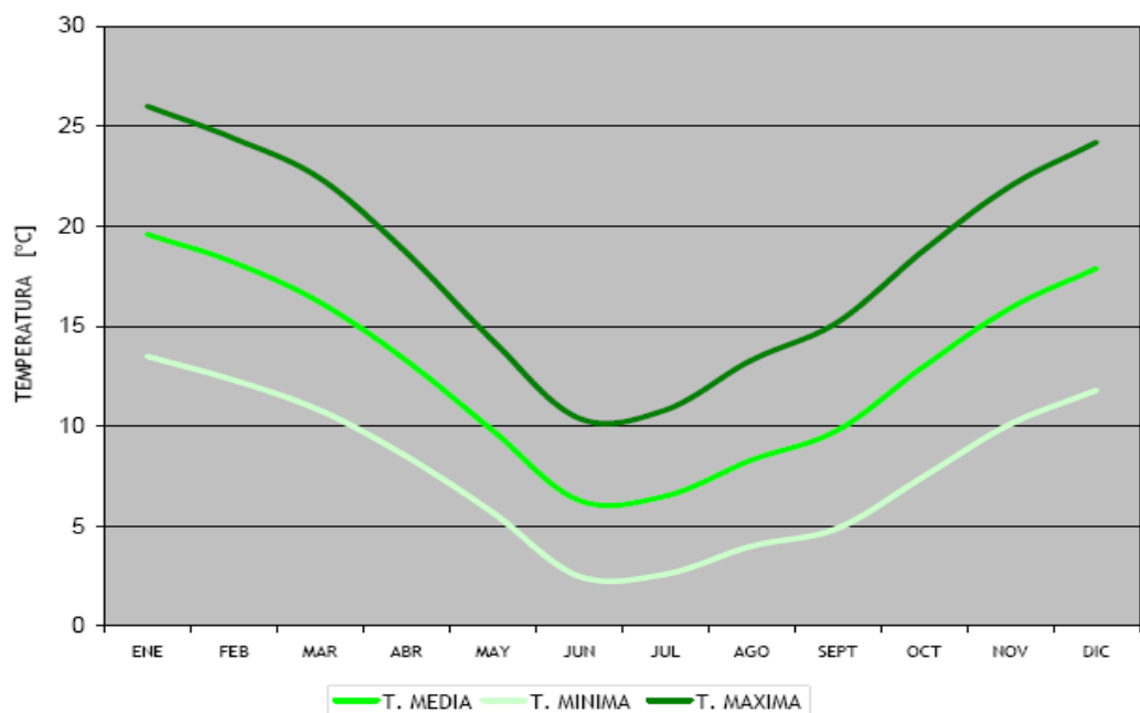
Figura 01. Variación mensual de temperaturas
