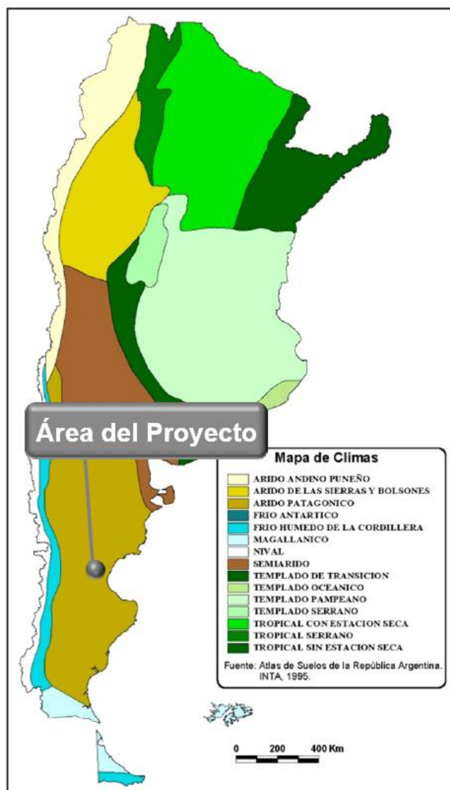
Mapa 01. Tipos de climas. Fuente.INTA
