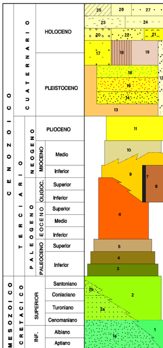
Figura 03 .Columna estratigráfica extraída de la Fuente. Hoja Geológica 4569-IV Escalante.
