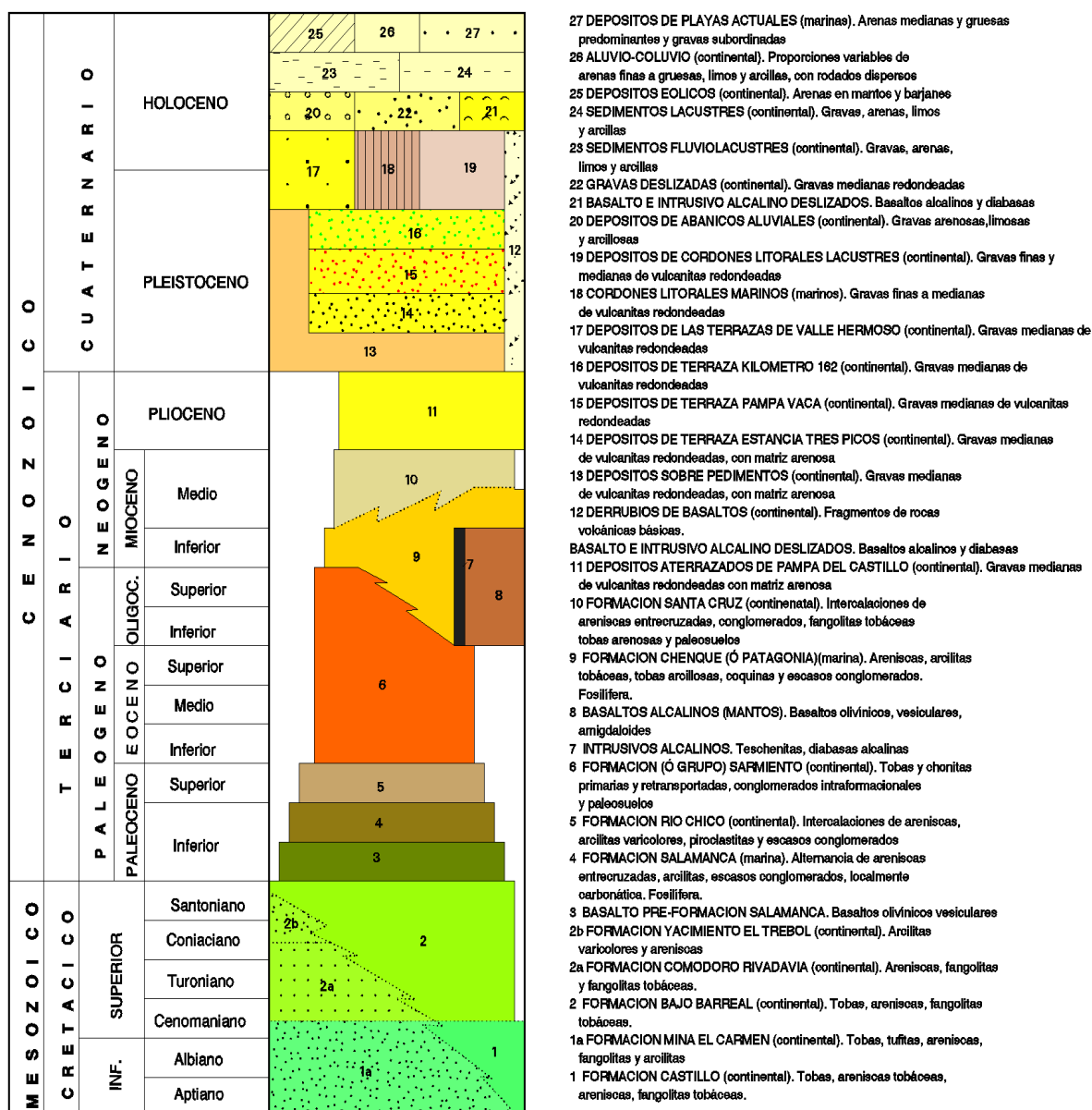
Figura 03. Columna estratigráfica extraída de la Fuente. Hoja Geológica 4569-IV Escalante.
