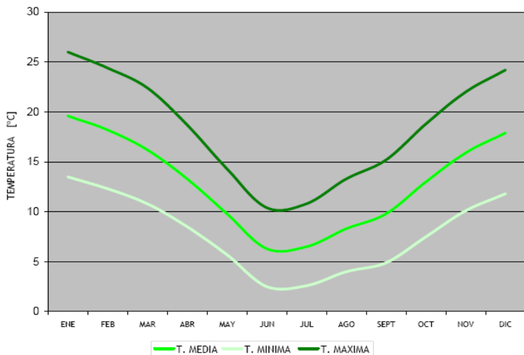
Figura 03. Variación mensual de temperaturas
