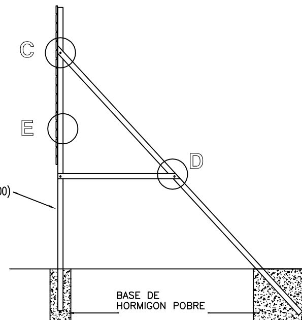
VISTA LATERAL
