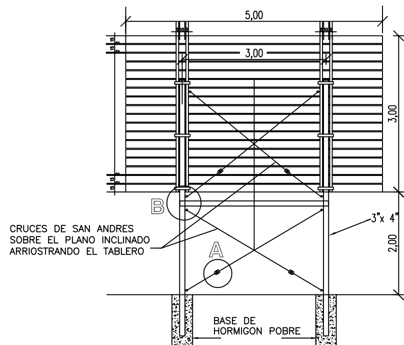
VISTA POSTERIOR
