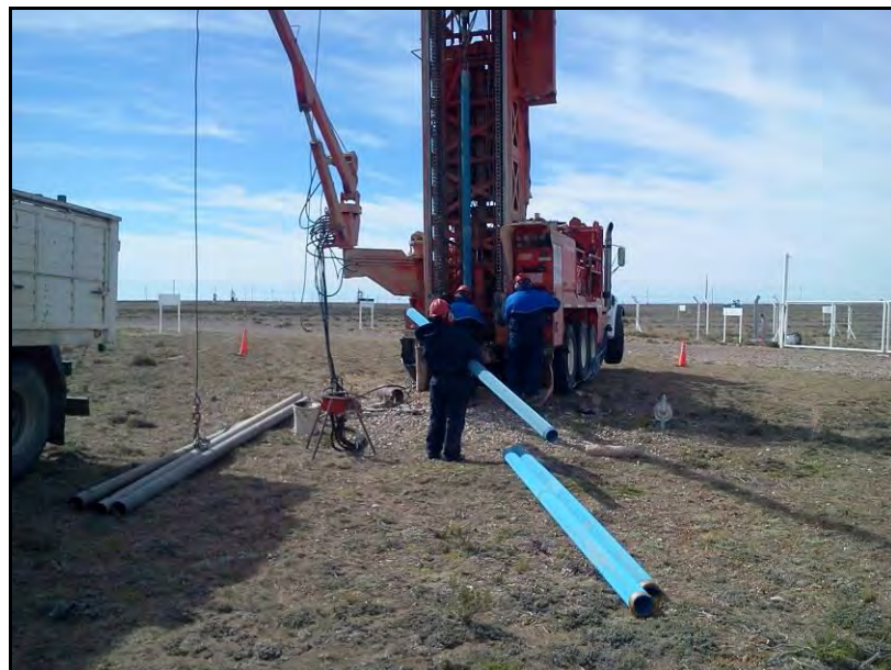
FOTO 6: Tarea de entubado utilizando cañería de PVC de 4 pulgadas.
